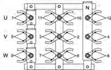
Connexion étoile serie + neutre
