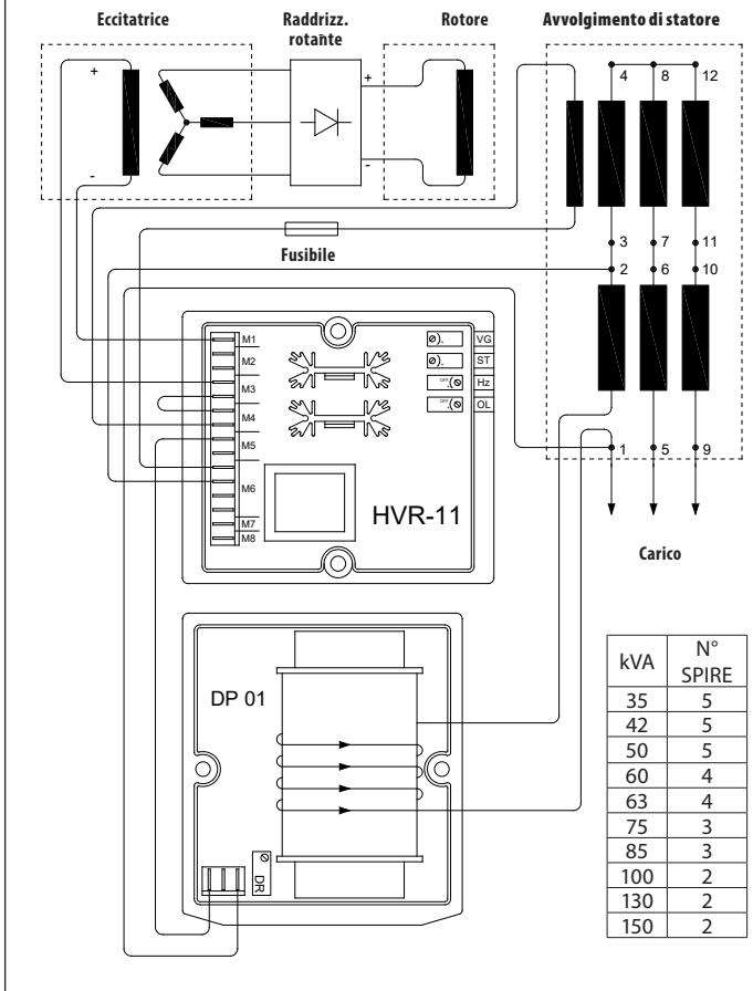
Fig. 17 - COLLEGAMENTO DEL DP01 CON IL REGOLATORE HVR-11
