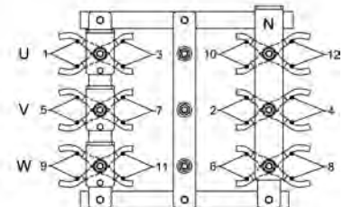
Connexion étoile parallèle + neutre
