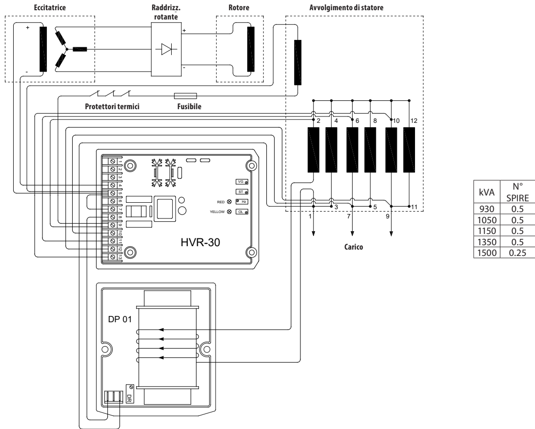
Fig. 20 - COLLEGAMENTO DEL DP01 CON IL REGOLATORE HVR-30 CON RIFERIMENTO DI TENSIONE TRIFASE (PRO 40)
