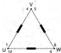
Треугольное соединение
