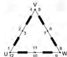
Сериальное треугольное соединение
