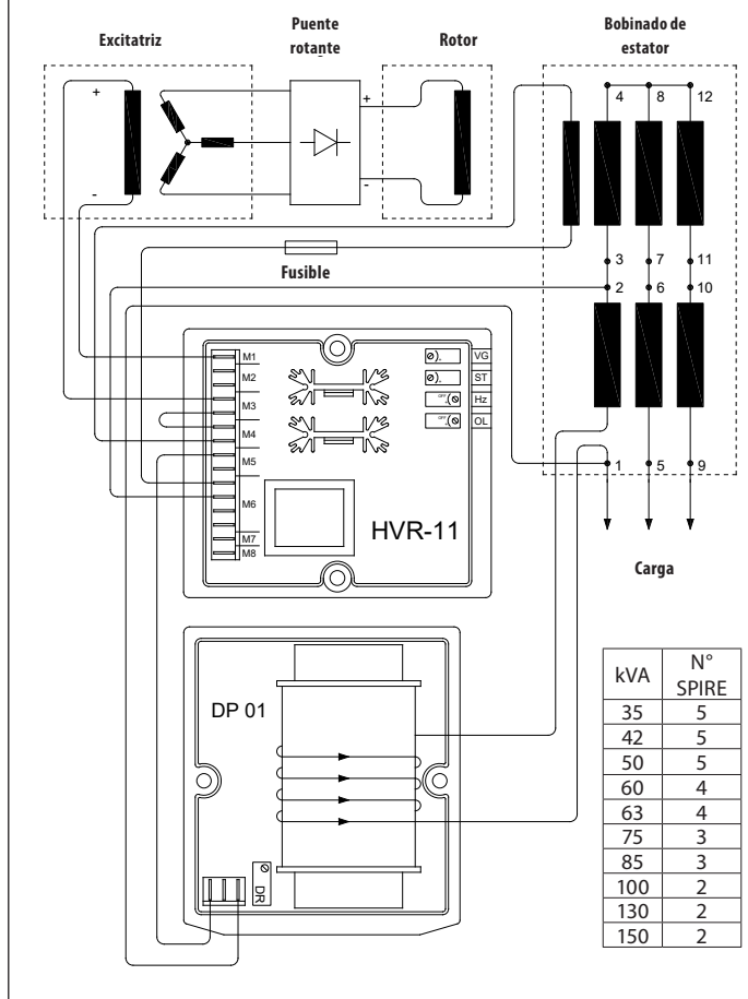
Fig. 17 - CONEXIÓN DEL DP01 CON EL REGULADOR HVR-11
