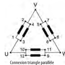
Connexion triangle parallèle
