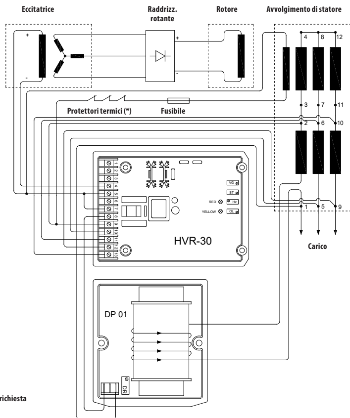
Fig. 19 - COLLEGAMENTO DEL DP01 CON IL REGOLATORE HVR-30 CON RIFERIMENTO DI TENSIONE TRIFASE (PRO 35)
