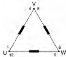
Connexion triangle
