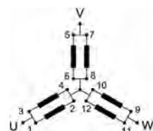
Параллельное + нейтральное соединение
