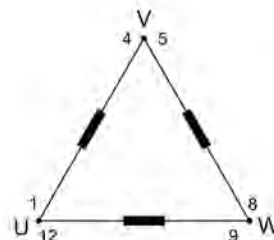
Connexion triangle
