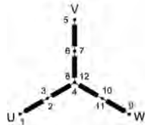
Connexion étoile serie + neutre
