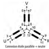
Connexion étoile parallèle + neutre
