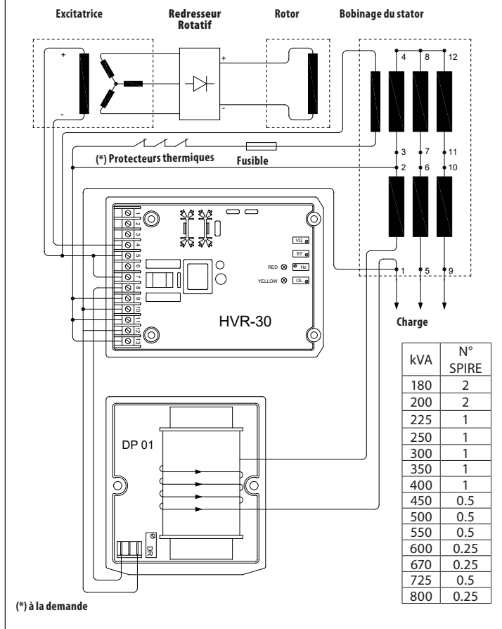
Fig. 18 - Connexion du DP01 avec le régulateur HVR-30 avec référence de tension monophasé
