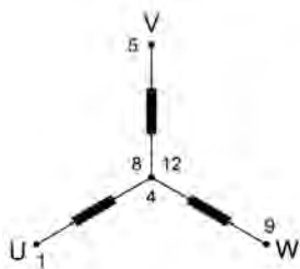
Connexion étoil+neutre
