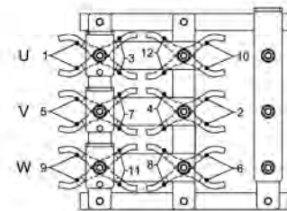
Connexion triangle parallèle
