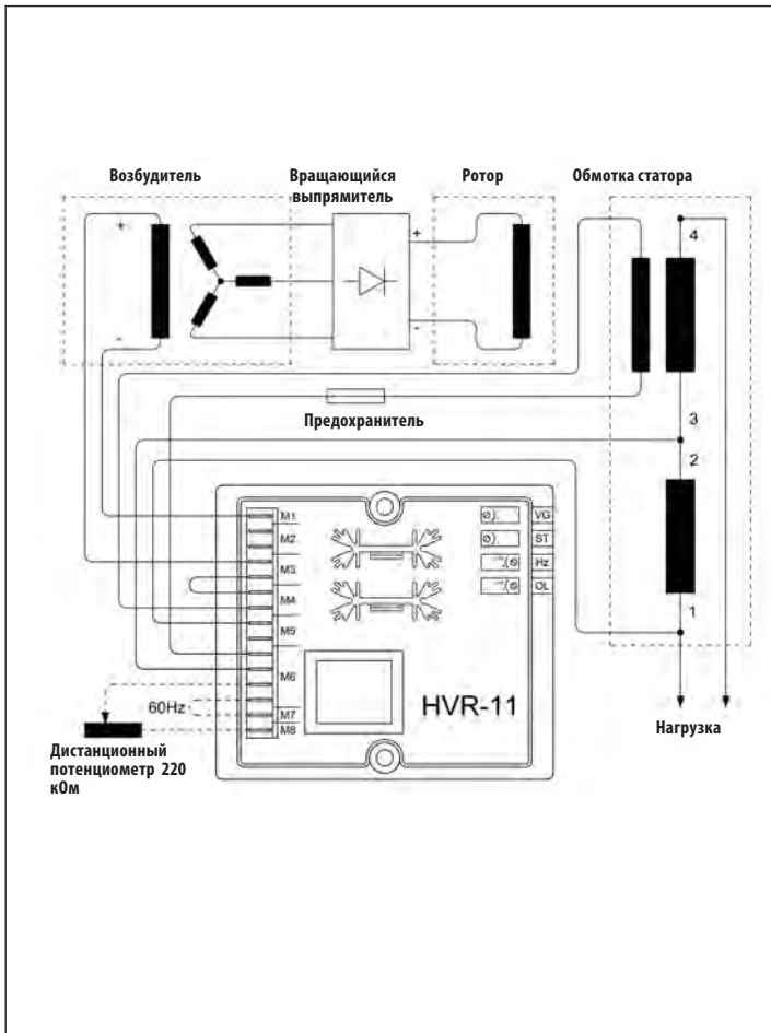
15 - ЭЛЕКТРИЧЕСКАЯ СХЕМА SLS
