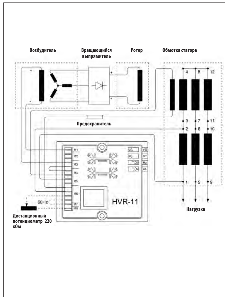
14 - ЭЛЕКТРИЧЕСКАЯ СХЕМА SLT - PRO 18 - PRO 22
