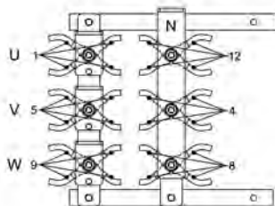
Звезда + нейтральное соединение
