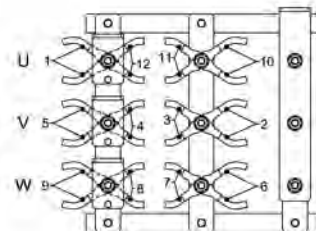
Сериальное треугольное соединение
