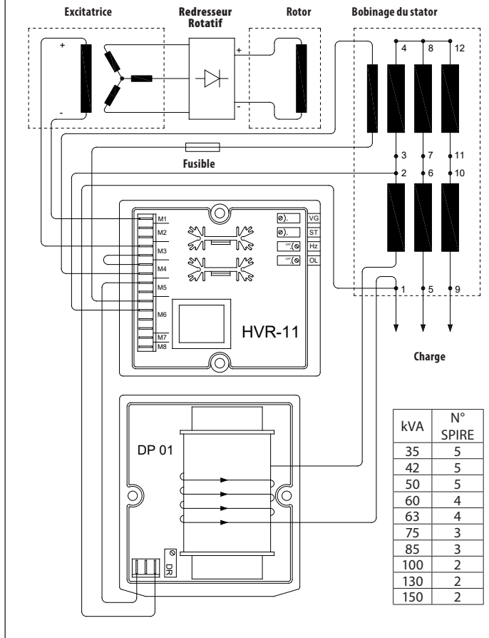
Fig. 17 - Connexion du DP01 avec le régulateur HVR-11
