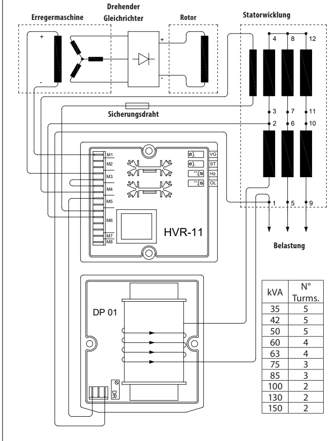
Abb. 17 - DP01 ZUSAMMENHANG MIT DER REGLER HVR-11
