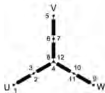
Соединение звезда + нейтральное соединение
