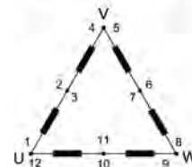
Delta serie connection 230 V - 50 Hz 276 V - 60 Hz
