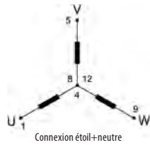
Connexion étoil+neutre
