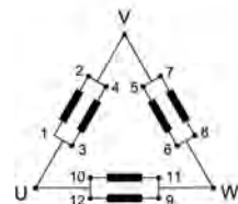
Параллельное треугольное соединение
