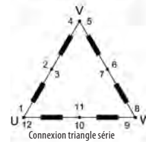
Connexion triangle série
